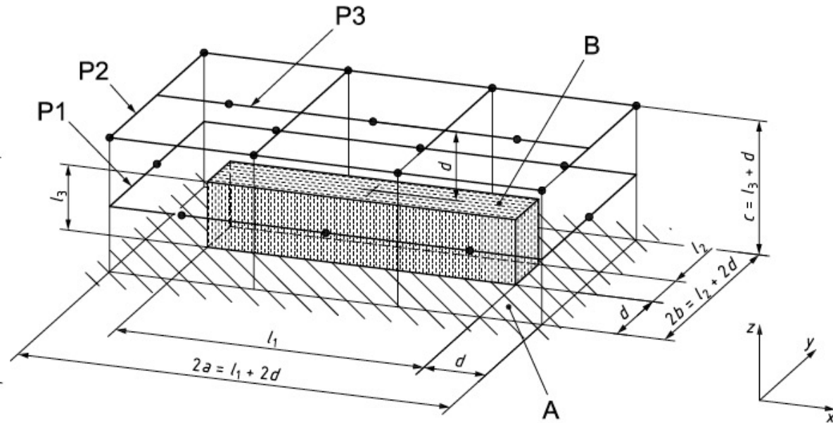
Superficie de medición con posiciones de sonómetros y caminos para una máquina larga
